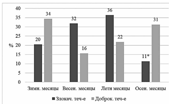
Рисунок 2. Тип течения и время рождения пациентов
